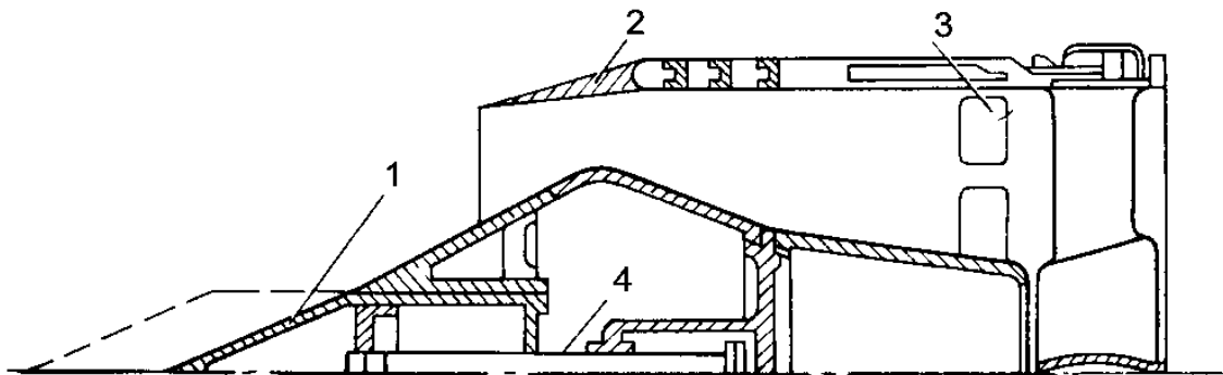
Рис. 2.2. Схема регулируемого СВУ внешнего сжатия:
