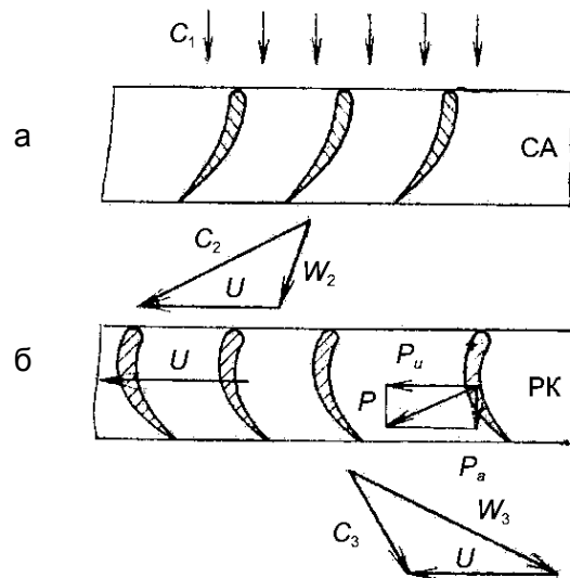
Рис. 5.2. Решетки профилей лопаток СА и РК
