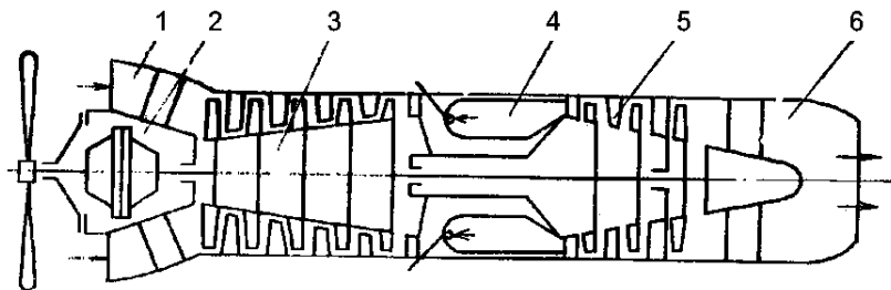
Рис. 1.5. Схема ТВД:
