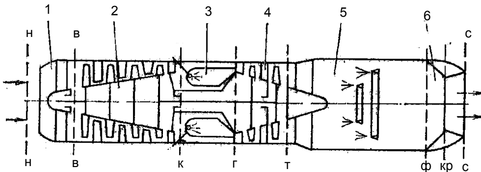
Рис. 1.3. Схема ТРДФ:
