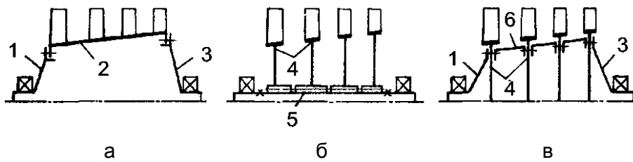
Рис. 3.3. Типы роторов ОК:
