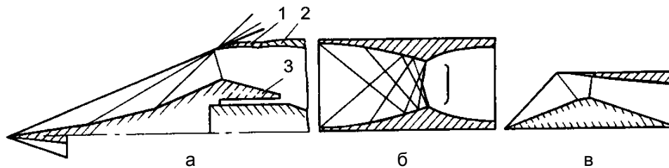
Рис. 2.1. Схемы сверхзвуковых диффузоров:
