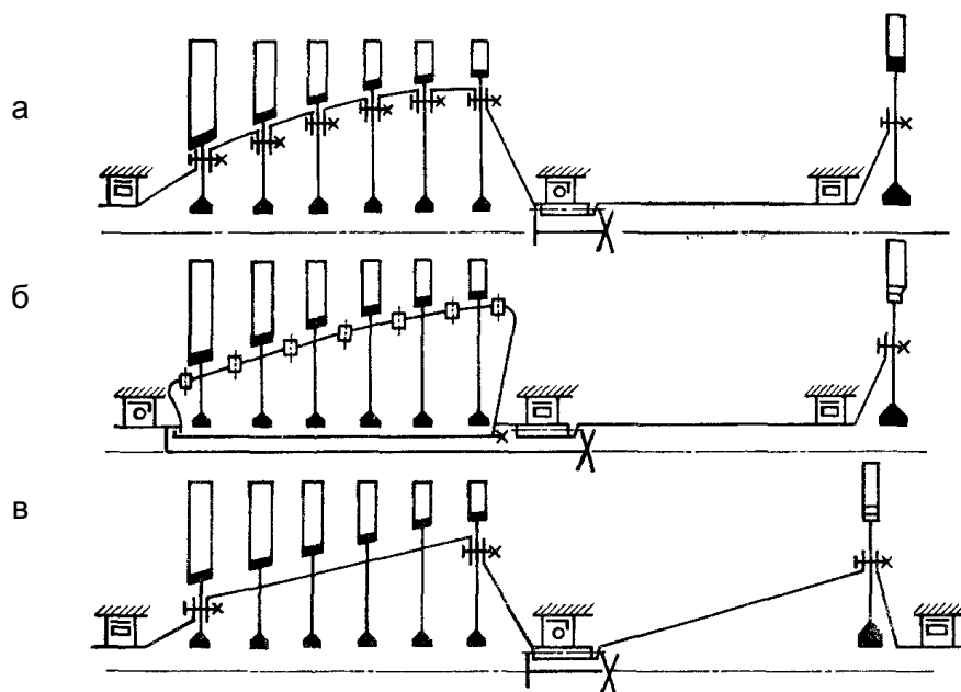
Рис. 1.8. Схемы трехопорных роторов с передним (а, б) и задним (в) расположением подшипника турбины
