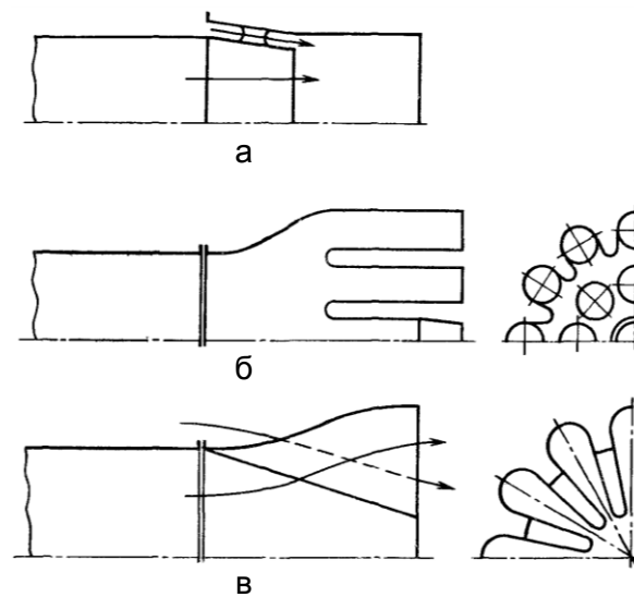
Рис. 6.7. Принципиальные схемы шумоглушителей на выходе ГТД: а – эжекторное сопло; б – многотрубное сопло; в – гофрированное сопло
