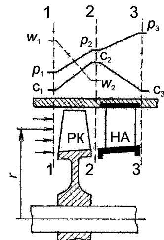
Рис. 3.1. Схема ступени ОК
