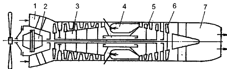
Рис. 1.6. Схема ТВД со свободной турбиной:
