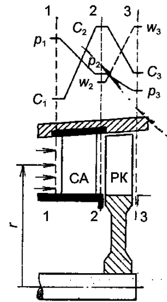
Рис. 5.1. Схема ступени ГТ
