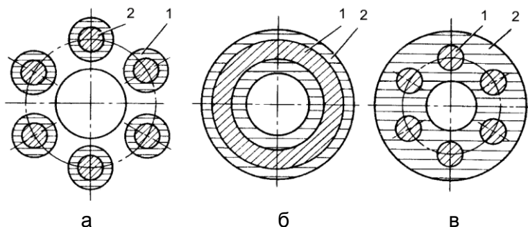
Рис. 4.1. Схемы КС:
